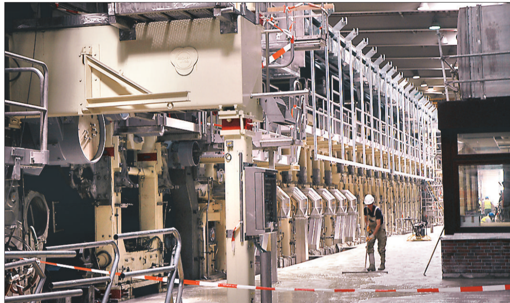
In Rekordzeit aufgebaut: die Papiermaschine 4 in Varel
